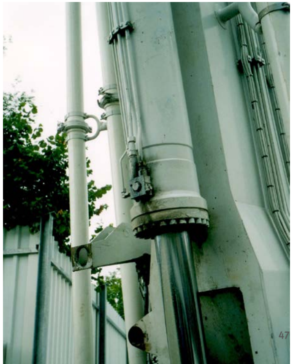
Abb. 18 Hydraulikzylinder mit entsperrbarem Rückschlagventil
